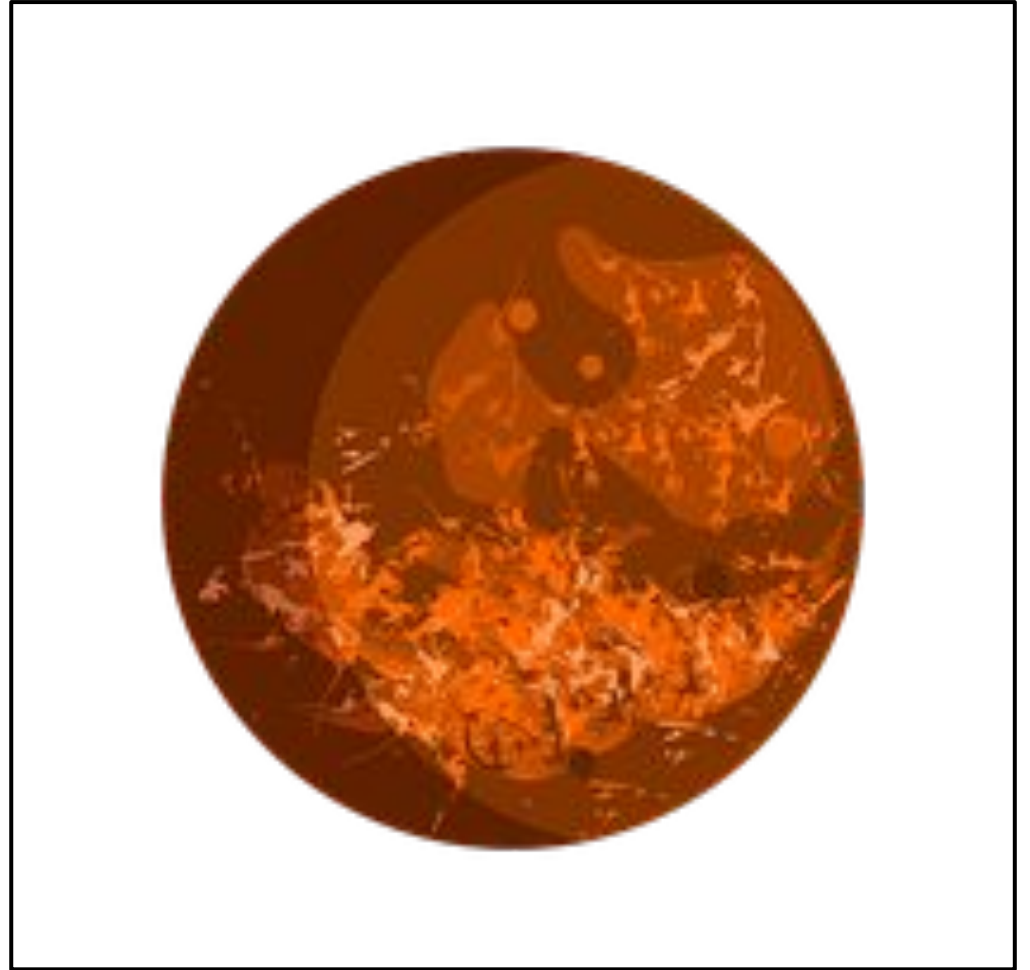
VENUS
