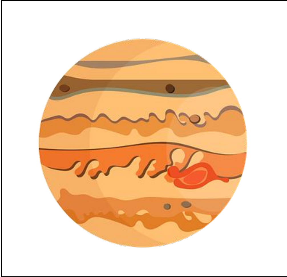
JUPITER
